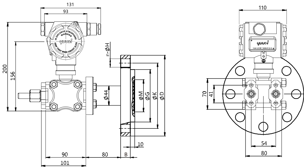
标准型扁平式不带显示机能的整机尺寸图
