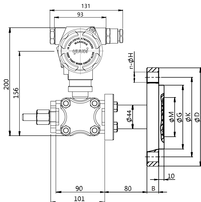
双隔膜型扁平式不带显示机能的整机尺寸图
