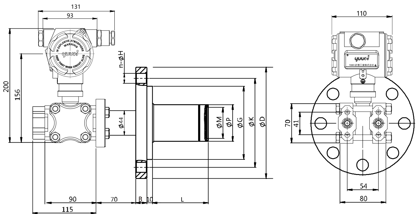
标准型插入筒式不带显示机能的整机尺寸图
