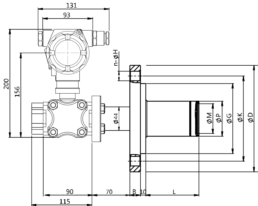
标准型插入筒式带显示机能的整机尺寸图（配A2接头）
