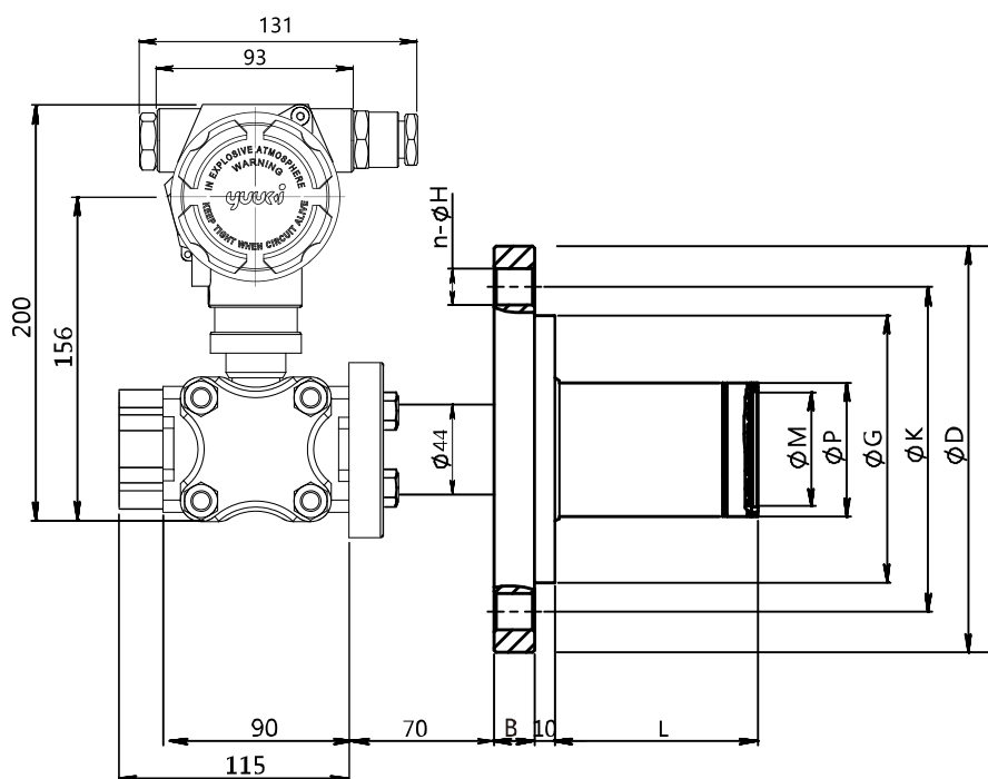
双隔膜型插入筒式不带显示机能的整机尺寸图
