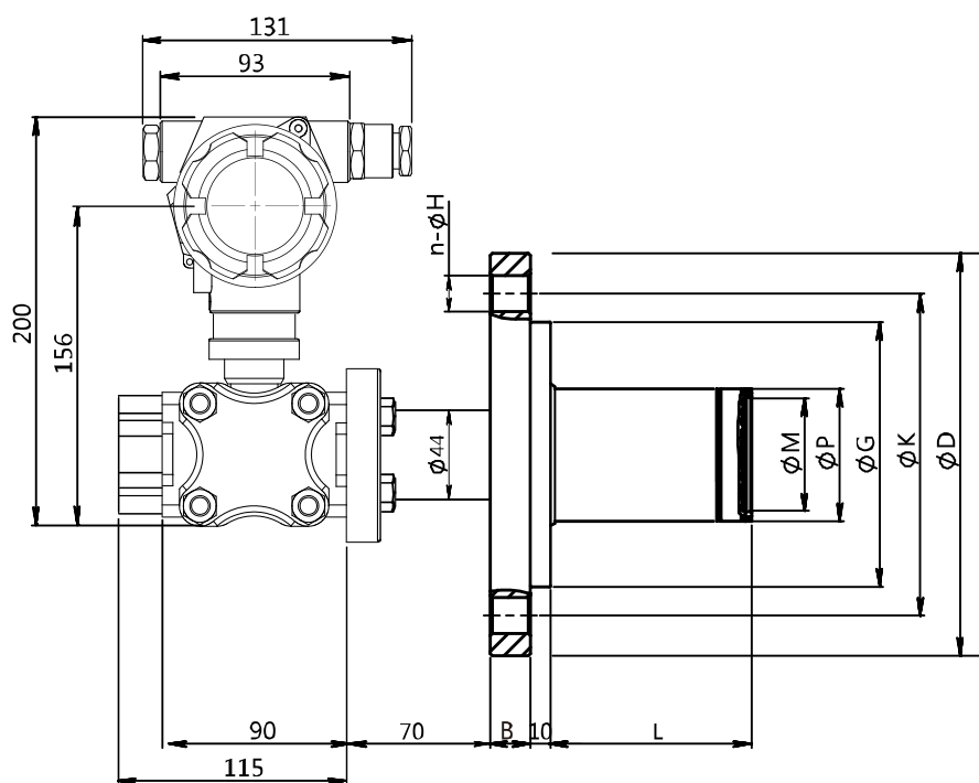
双隔膜型插入筒式带显示机能的整机尺寸图
