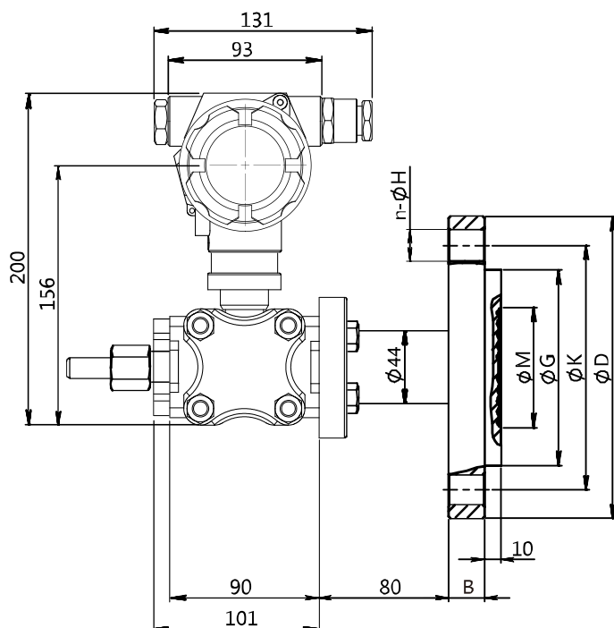
标准型扁平式带显示机能的整机尺寸图 (配A1接头)
