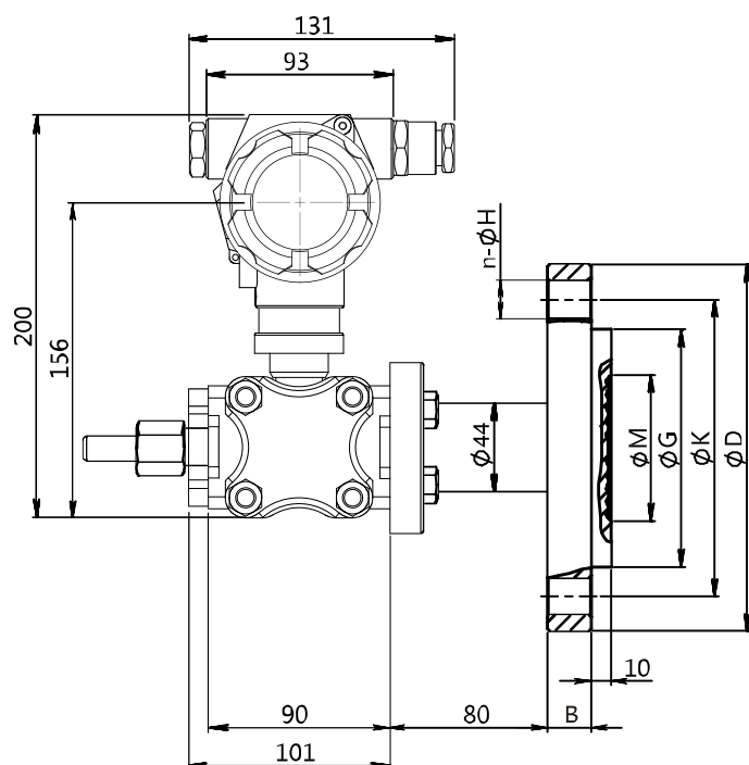
双隔膜型扁平式带显示机能的整机尺寸图
