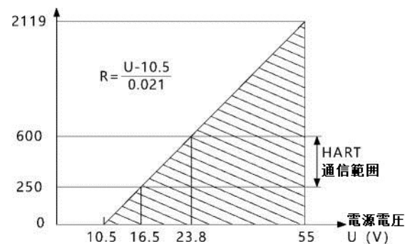
図 1 電源及び負荷条件
