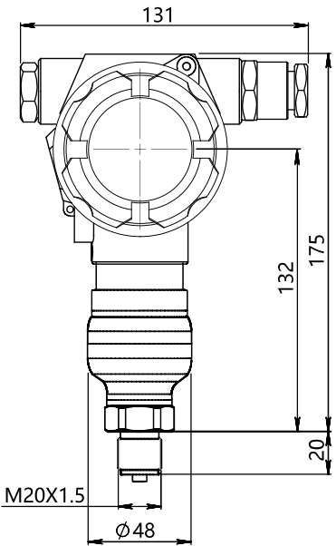
JUN-E20-H带显示机能的整机尺寸图
