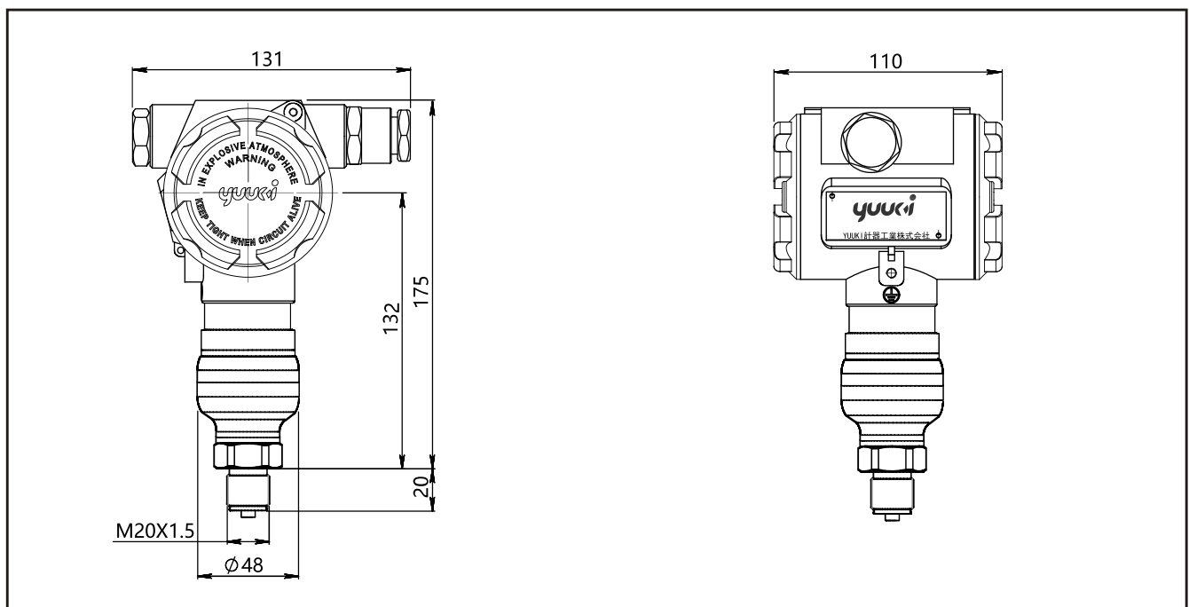
JUN-E20-H不带显示机能的整机尺寸图
