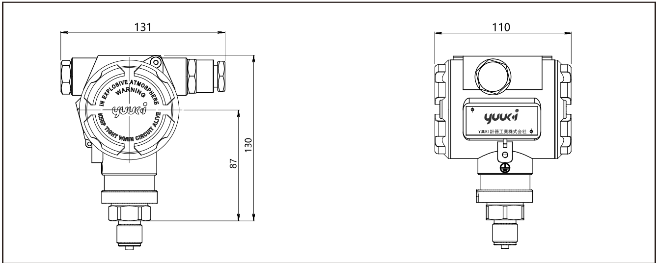
JUN-E20-S不带显示机能的整机尺寸图
