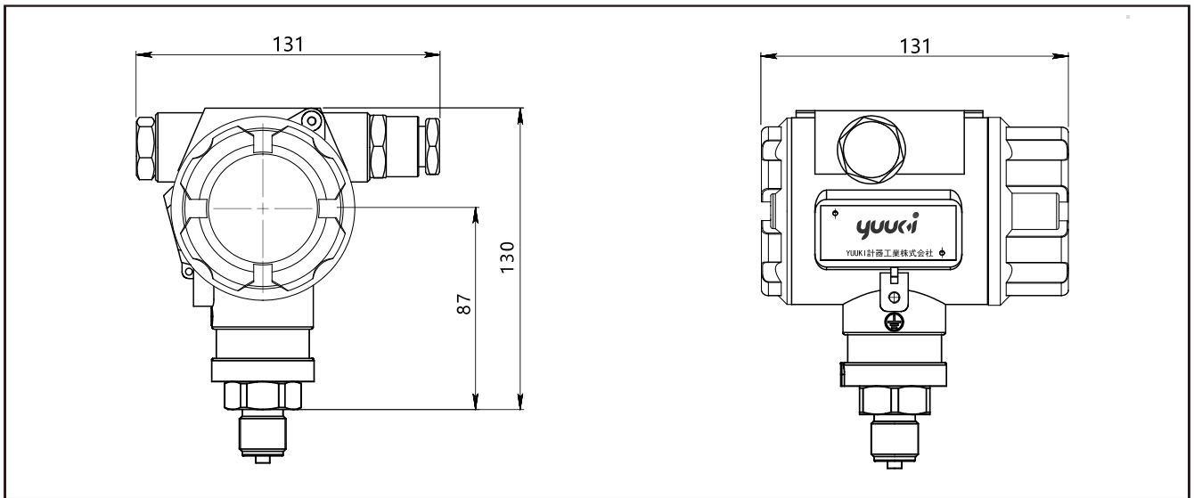
JUN-E20-S带显示机能的整机尺寸图
