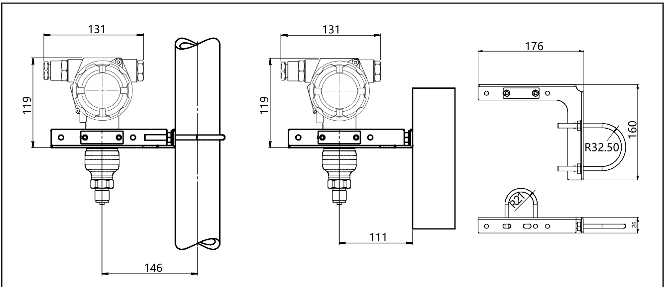
JUN-E20-H固定安装支架 (B4) 安装尺寸图
