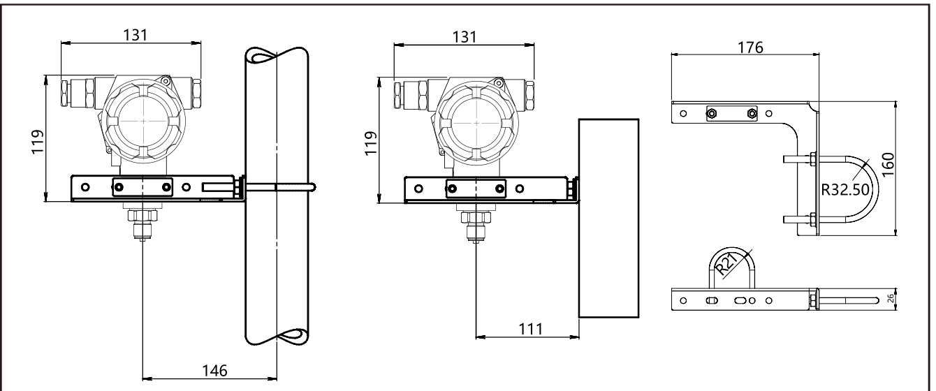
JUN-E20-S固定安装支架 (B4) 安装尺寸图
