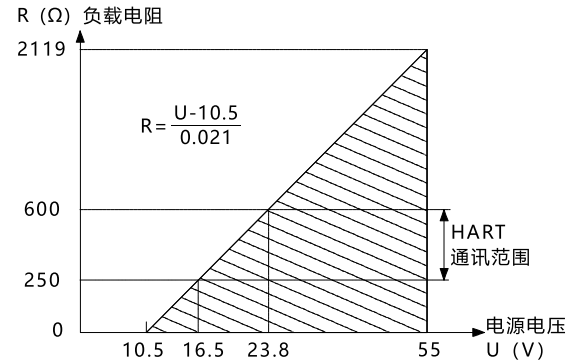
图1 电源及负载条件
